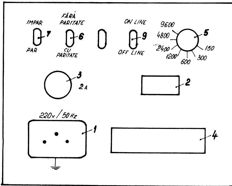
fig. 2.9.1. Panou spate
